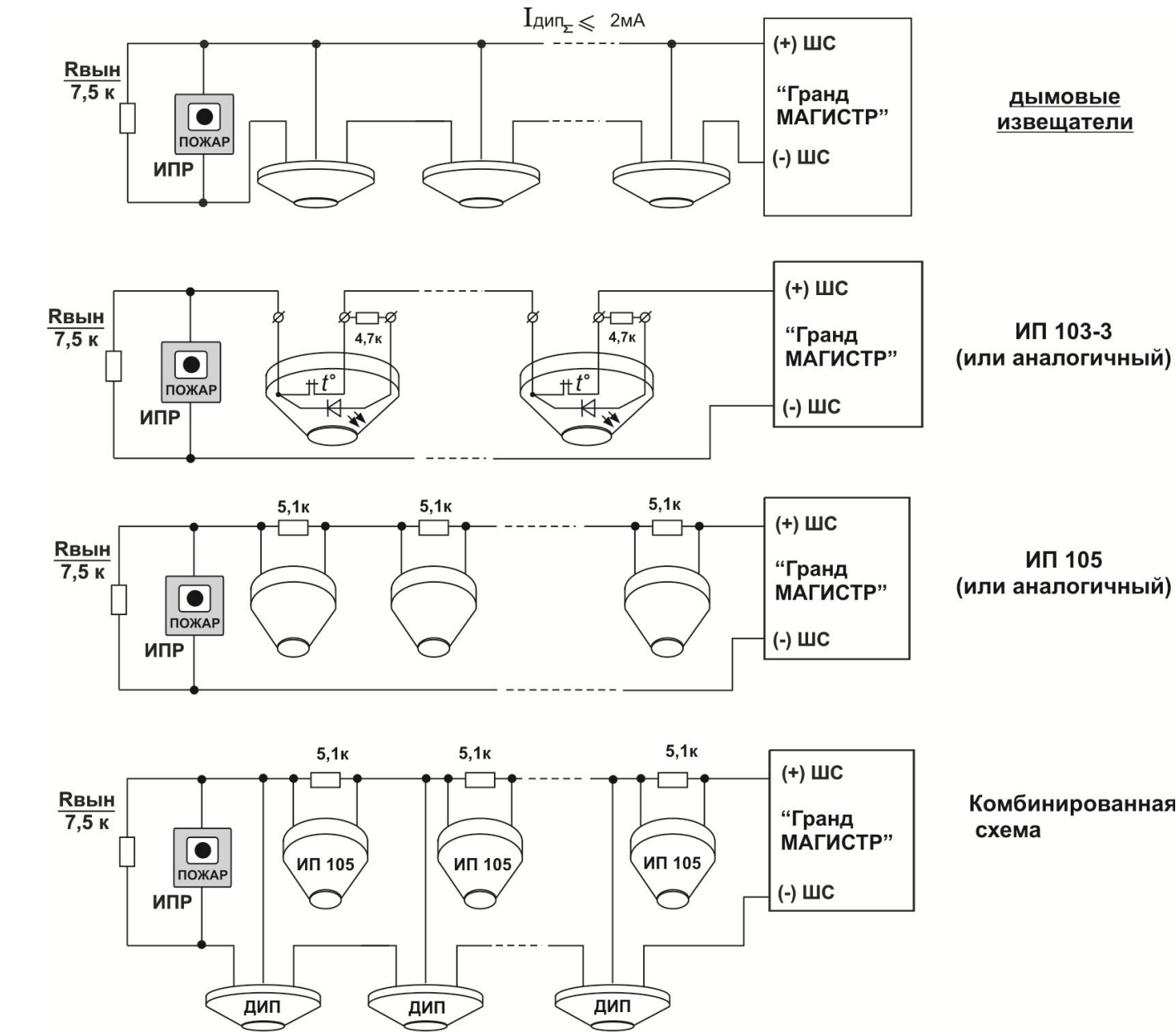
Рис. 8. Организация однопорогового шлейфа пожарной сигнализации
