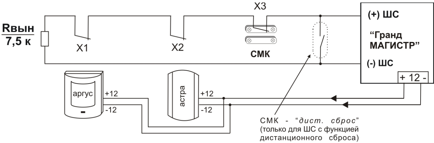
Рис. 8. Организация однопорогового шлейфа пожарной сигнализации
