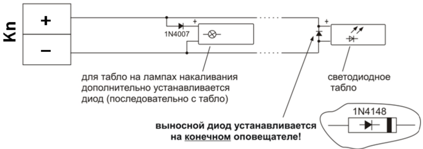
Рис. 10. Схема подключения нескольких световых табло
