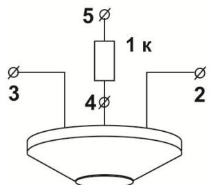
Рис. 12. Организация двухпорогового шлейфа пожарной сигнализации.
