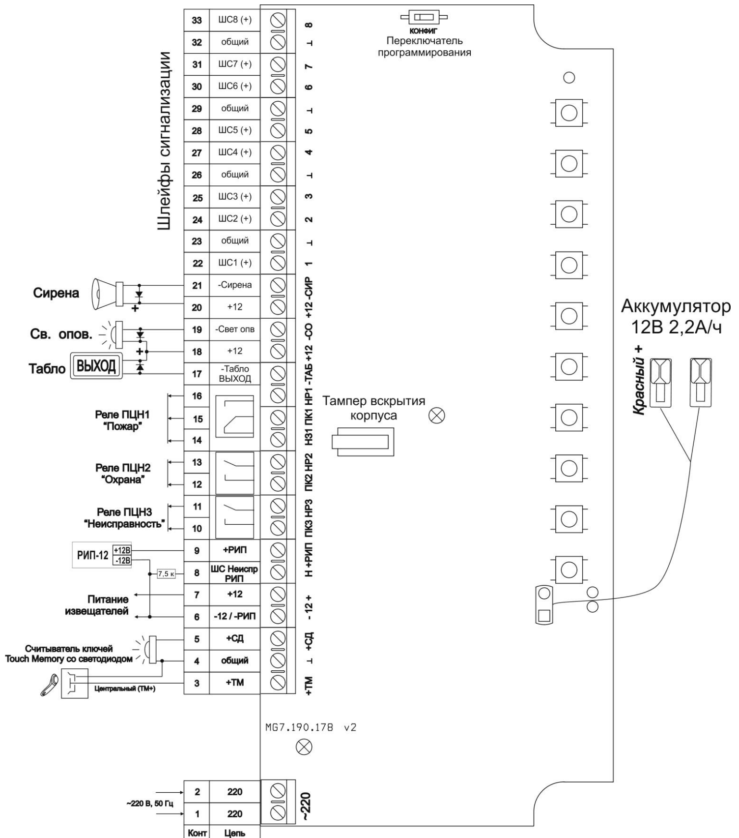
Рис. 2. Схема внешних соединений прибора Гранд МАГИСТР 8А (версия 2). Количество ШС зависит от исполнения прибора.
