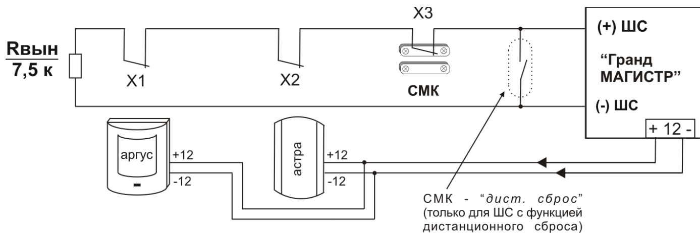
Рис. 5. Организация однопорогового шлейфа пожарной сигнализации
