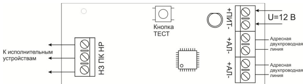
Рис. 1 Схема подключения УР.
